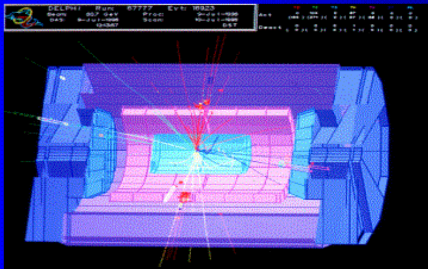
Ereignis mit W-Zerfall DELPHI (CERN, Genf), 1996
