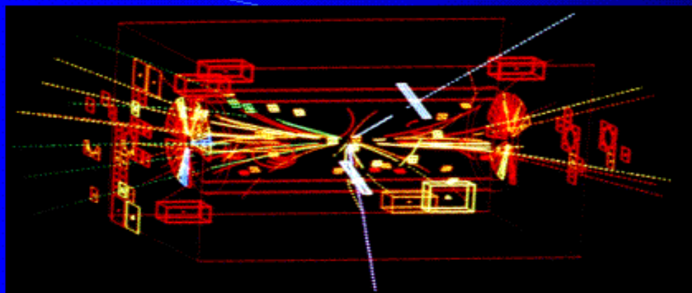
Ereignis mit W-Zerfall DELPHI (CERN, Genf), 1996
