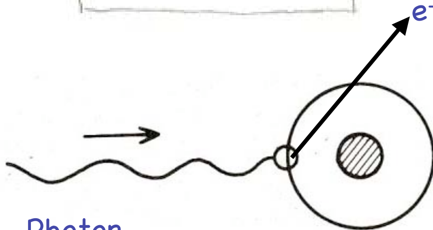
Atom mit Elektron
