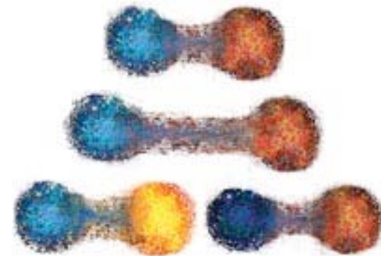
Quark-Antiquark Paare
