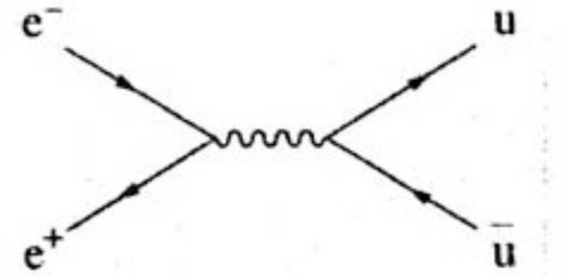
Quark-Antiquark Paare
