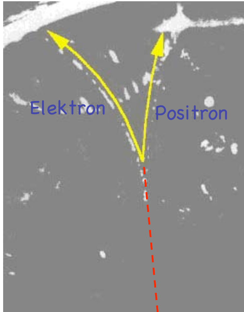
Ein Photon hoher Energie
