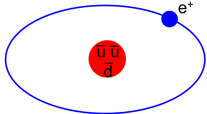
Antimaterie
