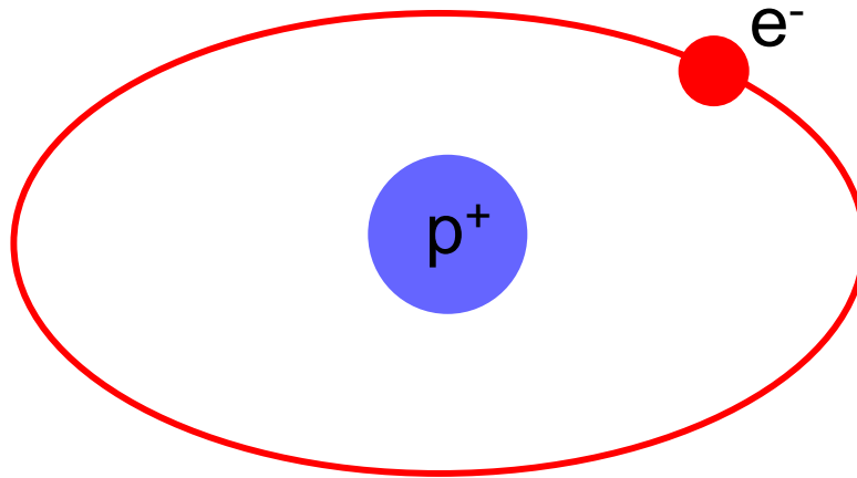
Materie
